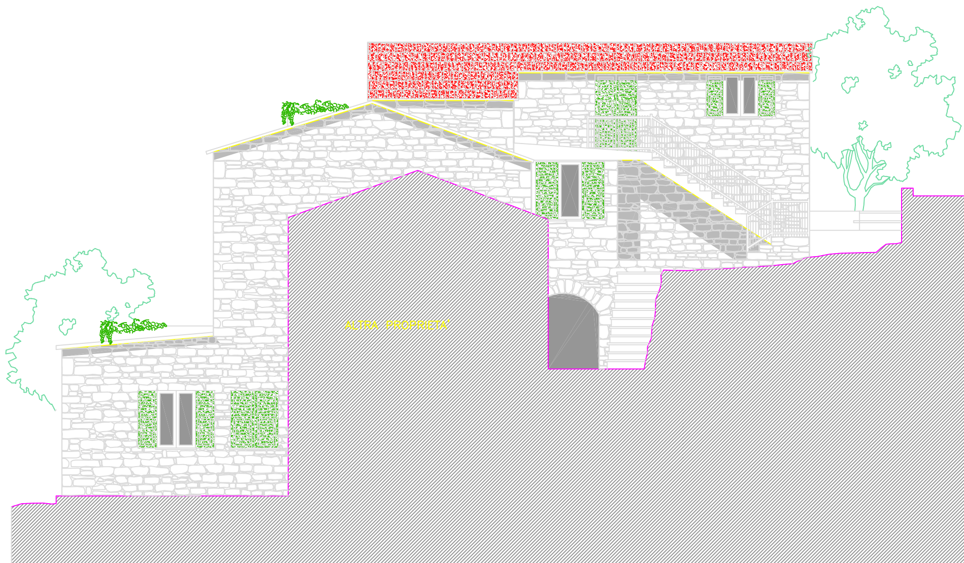
PROSPETTO OVEST
